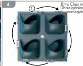
Beginnen Sie mit der linken oberen Ecke und drücken Sie einen Clip von Hand in den vorgesehenen Schlitz der Zelle. Verwenden Sie keinen Hammer o.ä.. Verwenden Sie Clips im Uhrzeigersinn verriegeln.
